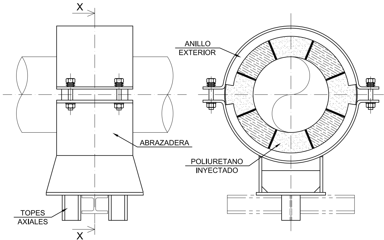
VISTA LATERAL
